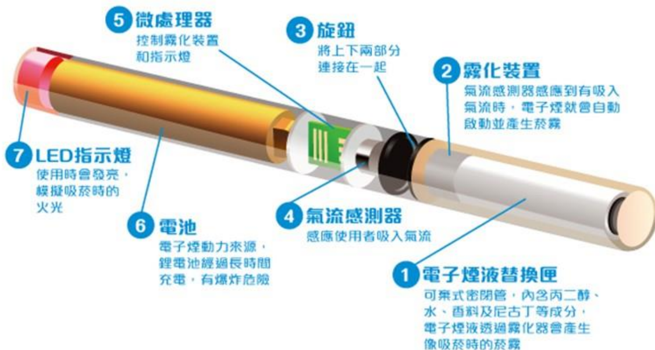
圖一：電子煙構造圖。引用自 董氏基金會華文戒菸網 。
